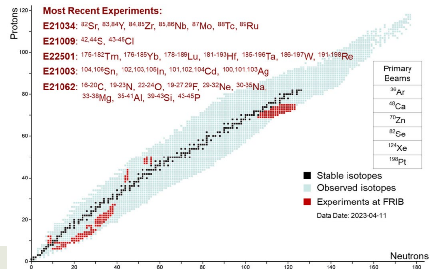
>200 unstable isotopes
